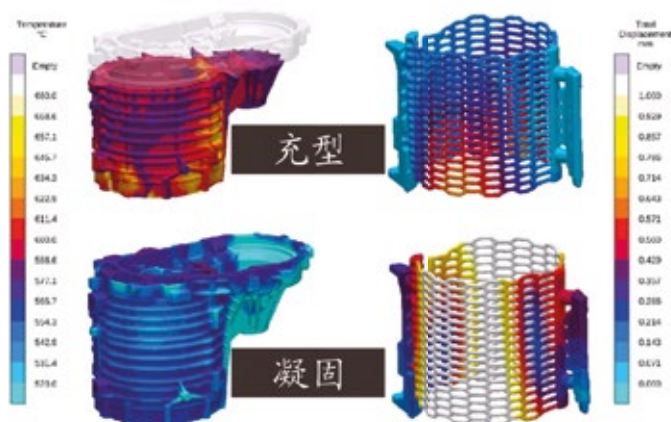
充型和凝固期间的砂芯变形
