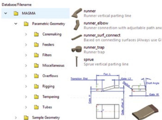
数据库中含有金属型铸造工艺所需的参数化几何
