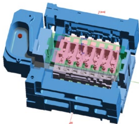
上图为详细的工艺模型，含铸模、滑块、砂芯或镶件以及复杂的冷却和加热管路。
