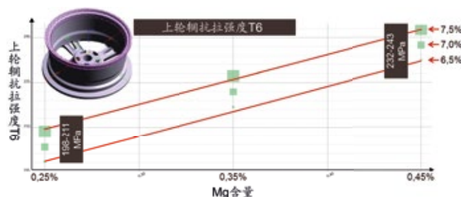
T6后Mg和Si的变量对抗拉强度的影响
