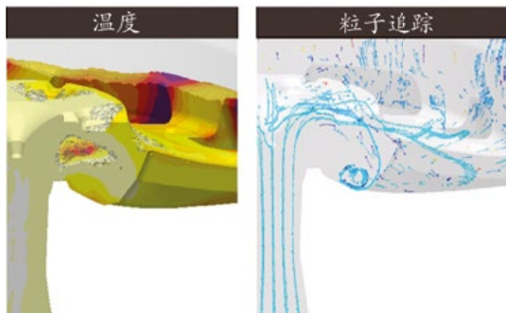
充型和潜在铸件缺陷的（如冷隔或氧化夹杂物）分析结果
